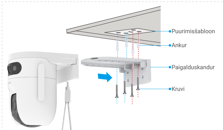
Joonis 1 Lakke kinnitamine
